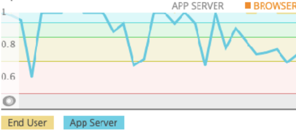
Apdex score
